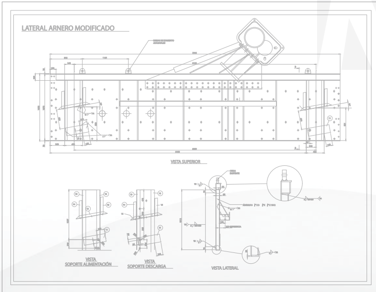
Planificación y rediseño de harnero lateral
